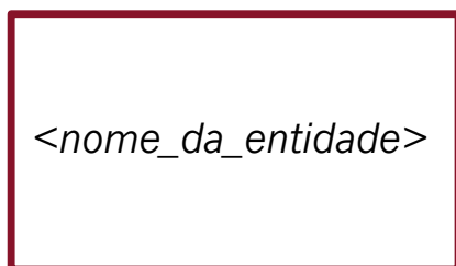
Entidade
