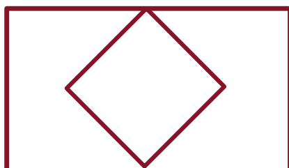
Entidade Relacionamento
