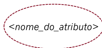
Atributo Derivado
