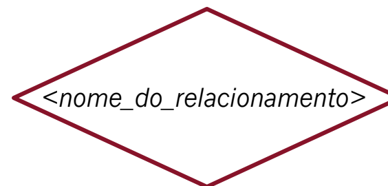
Relacionamento
